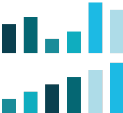
Fig. 5 Problème du tri. Des objets peuvent être triés selon une relation d'ordre, en lien avec une propriété. Sur la ligne du haut, les rectangles sont organisés selon leur couleur (de la plus sombre à la plus claire), alors que sur la ligne du bas, ils sont triés selon leur taille (du plus petit au plus grand).
