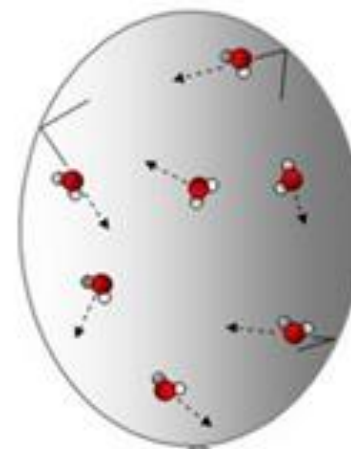
H 2 O(g)
