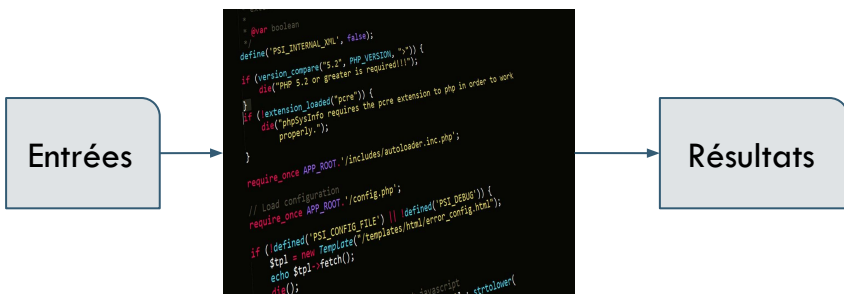
Programmation classique
