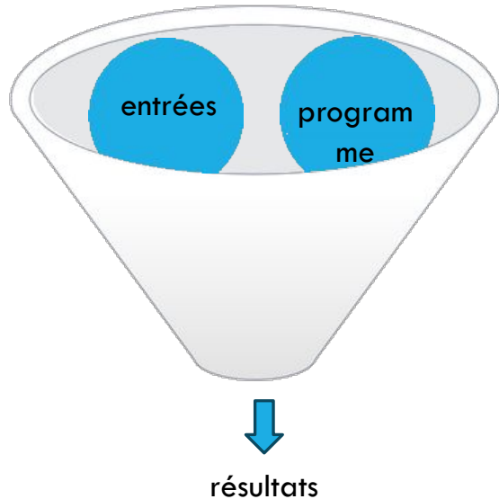
Programmation classique
